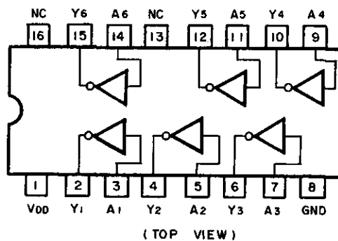
Fig. 13.8 Inverter C-MOS IC \mu PD4049BC
