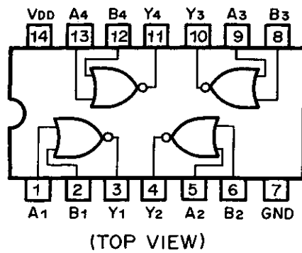
Fig. 13.9 NOR Gate C-MOS IC \mu PD4001BC
